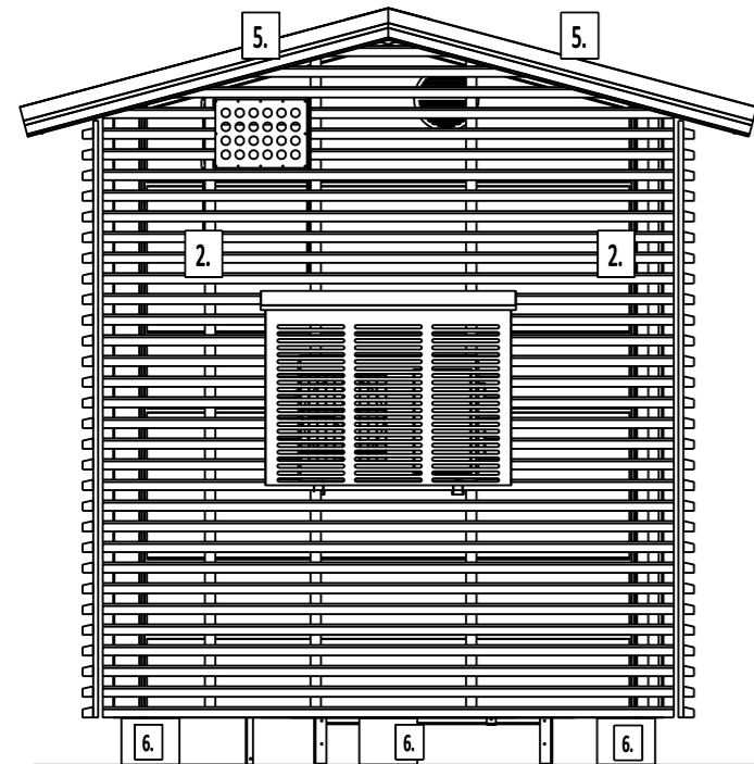
JULKISIVU C-D
