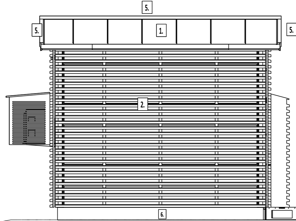
JULKISIVU B-C
