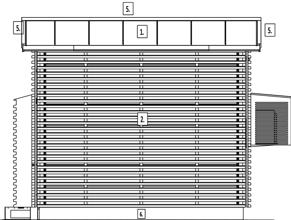
JULKISIVU D-A
